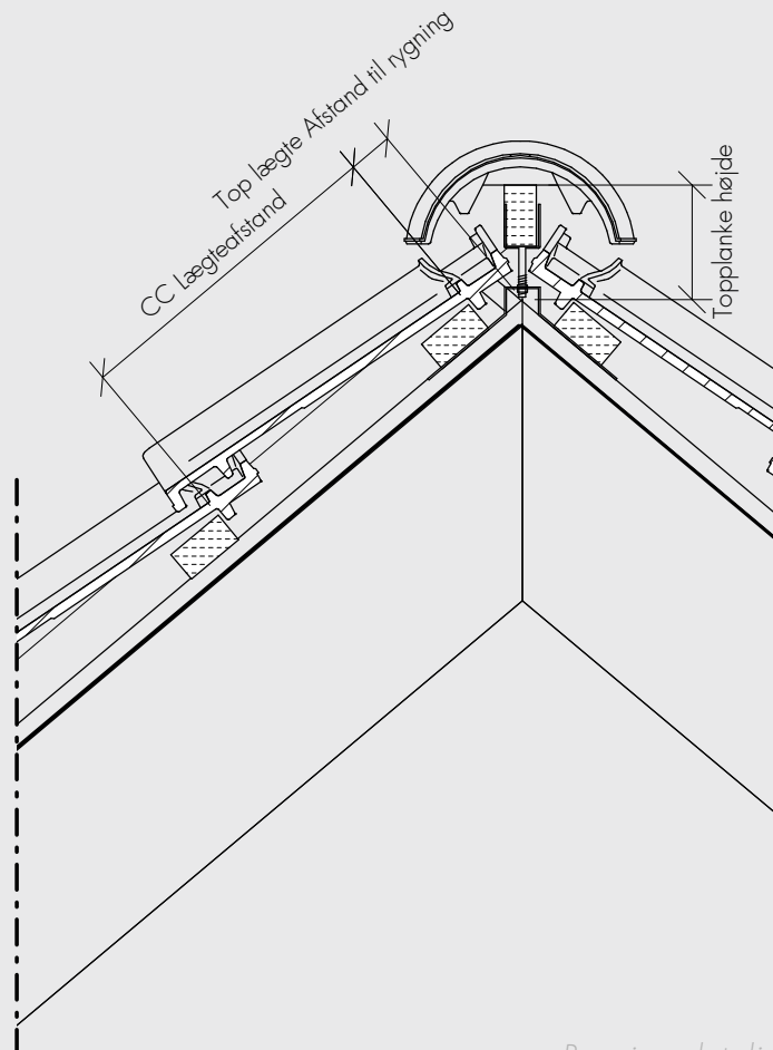
Rygningsdetalje
