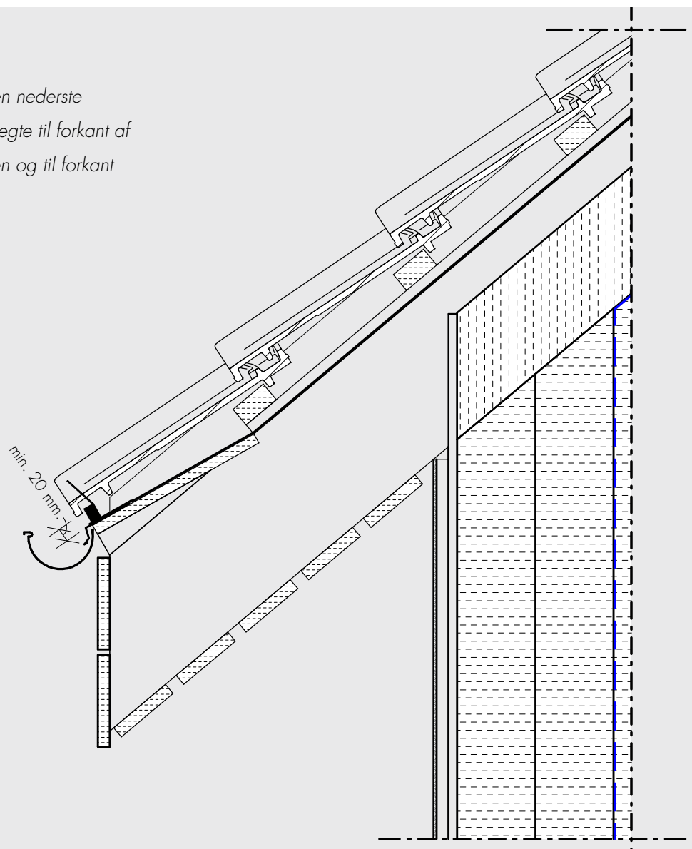
Tagfodsdetalje (let-konstruktion)
