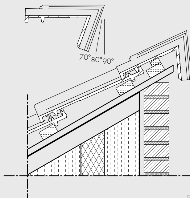
Rygningsdetalje
