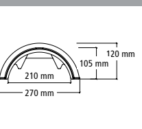
Konisk rygsten PKO (2,5 stk./m)
