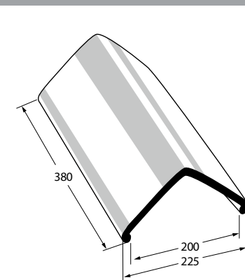
Samle Rygsten
