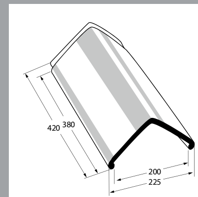
Vinkel rygsten 2,6 stk. pr. lbm.
