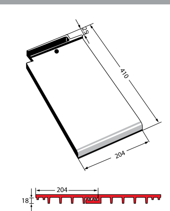
Dobbeltvinget
