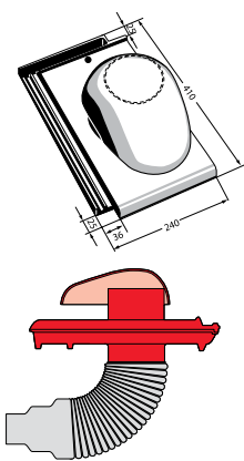
lodret tudsten ø 100 til 125 mm
