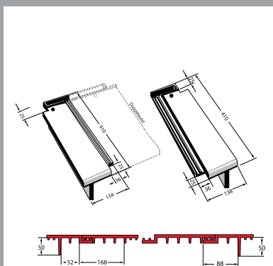
Halv vindskedesten højre & venstre
