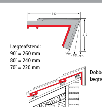
Pultsten
