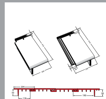
Vindskedesten højre & venstre
