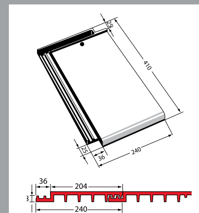
Almindelige tagsten
