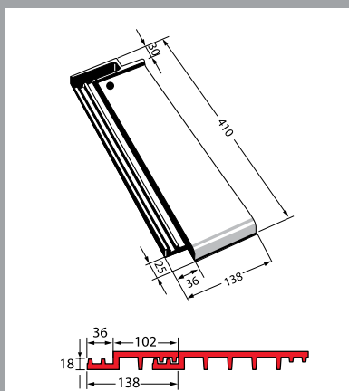
Halv tagsten
