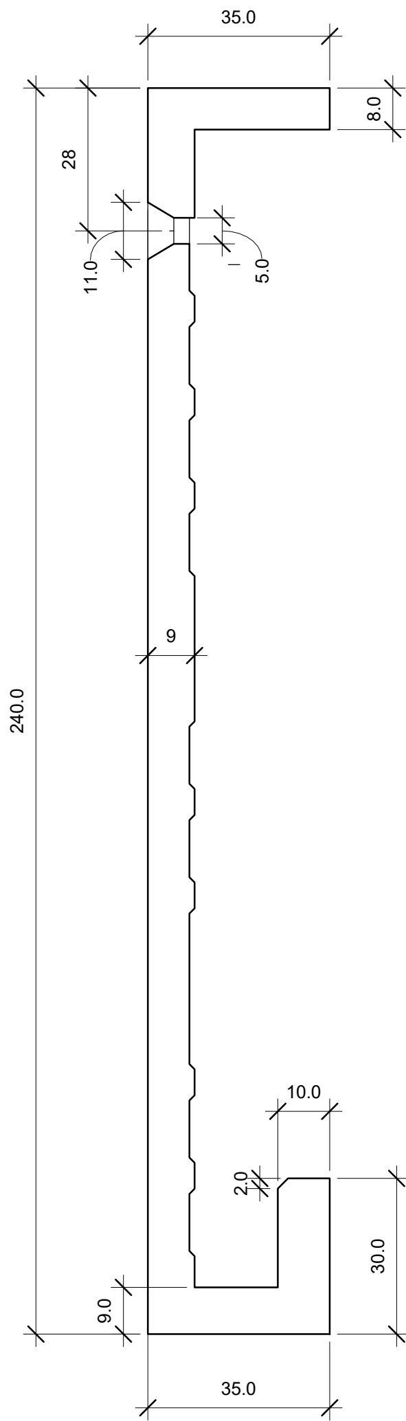
VERTICO RS U-shape skærmtegl
