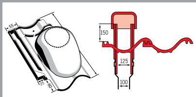
Lodret tudsten Ø100 til 125 mm
