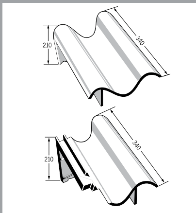
Pult / vindskedesten inde
