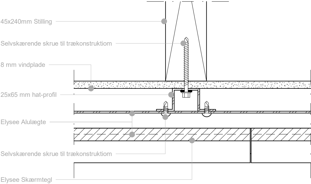
Vandret snit
