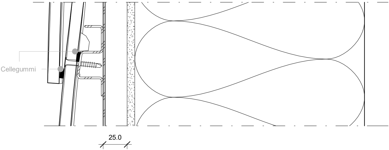
Lodret snit
